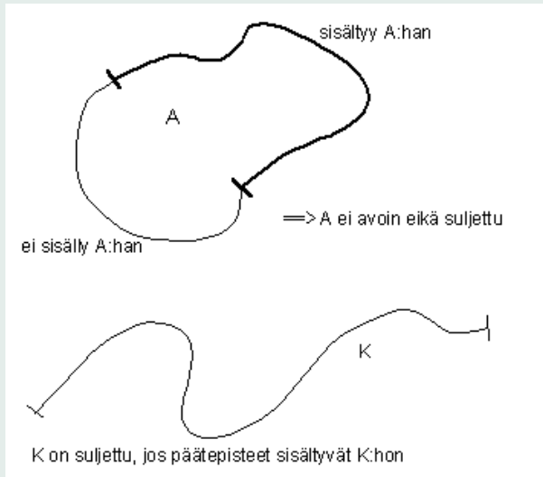
Kuva 8: Joukot A ja K
