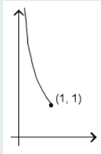
Kuva 12: käyrä f(t) := (t, \frac{1}{t})
