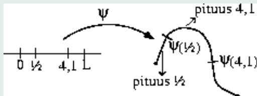
Kuva 26: Parametrisaatio polulle \Gamma
